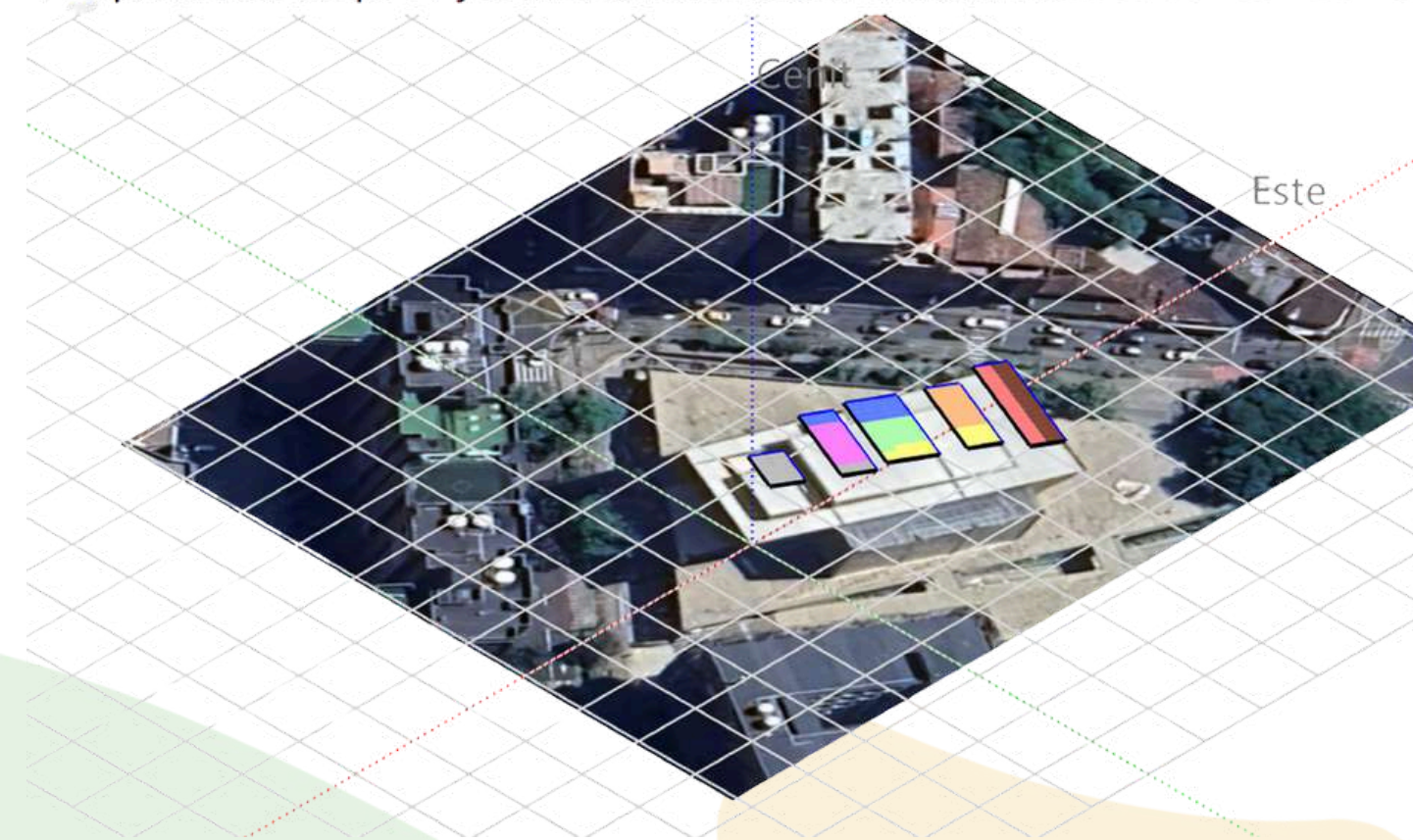
Perspectiva del campo FV y la escena de sombreado circundante
