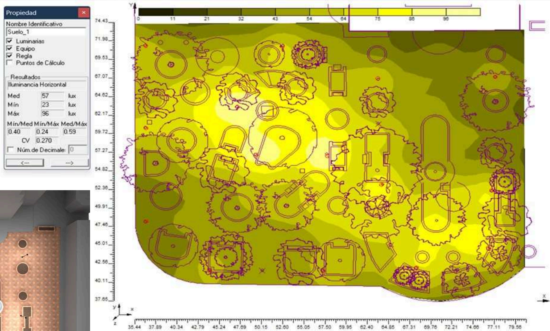
*Mapa luminotécnico
